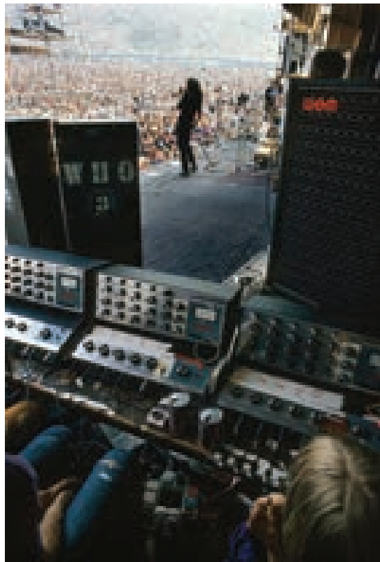
29 de agosto de 1970, 3er festival anual de la Isla de Wight, Sistema de PA de “The Who” y vista detallada de tres mezcladores WEM Audiomaster empleados para el multitudinario evento
