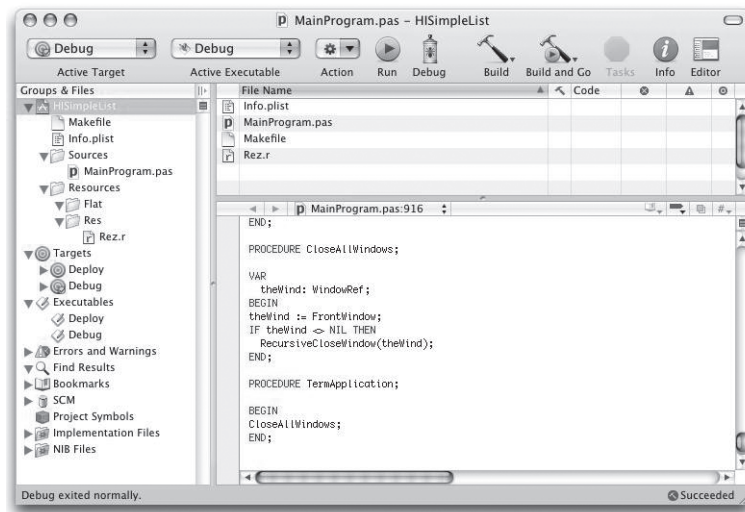
Figura 1.17. Herramientas Xcode
