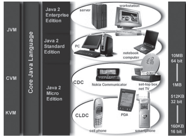
Figura 1.36. Entorno Java 2
