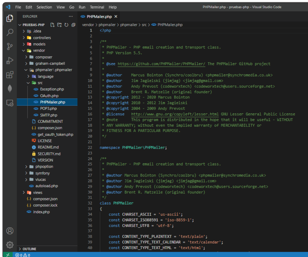
Figura 2.11. La carpeta vendor no debería commitearse, y contiene el código de las librerías instaladas con Composer.
