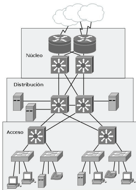
Modelo jerárquico de tres capas
