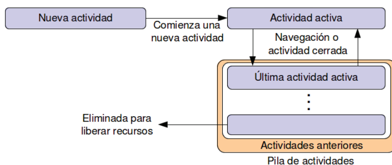
Figura 1.1. Diagrama de la pila de actividades
