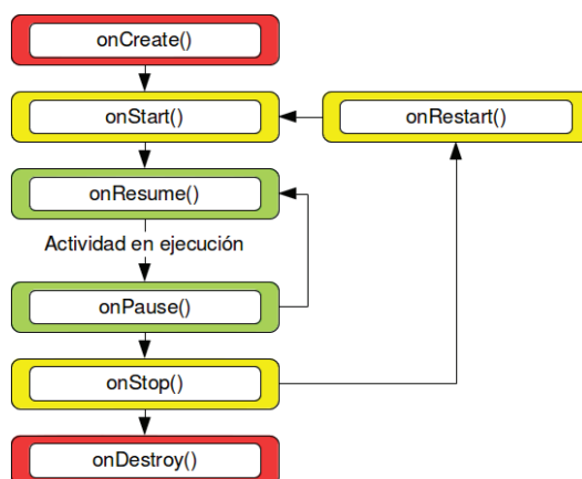
Figura 1.2. Ciclo de vida de una actividad
