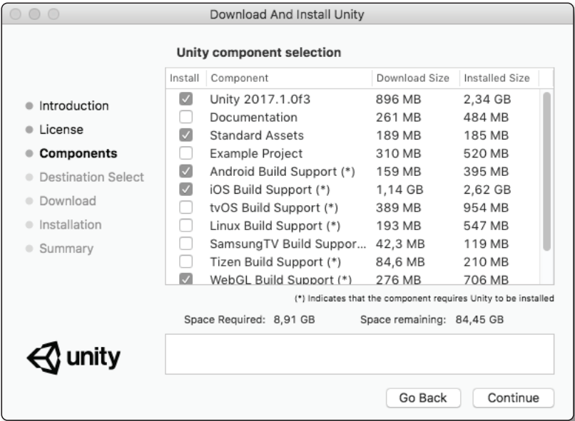
Figura 1.1. Opciones de instalación
