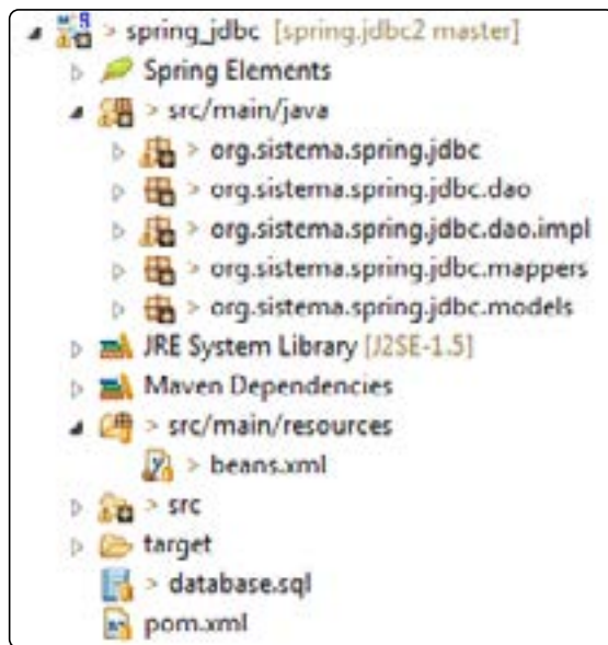
Figura 14.2. Estructura de un proyecto Spring
