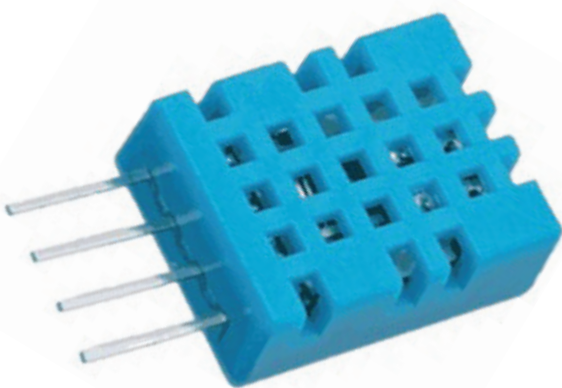
Figura 3.1. El sensor DHT11 tiene su carcasa de color celeste para diferenciarse de los otros modelos. Posee un rango de medición aceptable para ciertas aplicaciones. Como desventaja, no permite medir temperaturas bajo cero.
