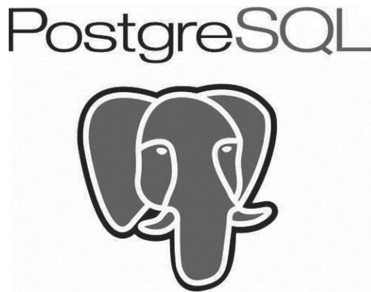
Figura 1.18. PostgreSQL
