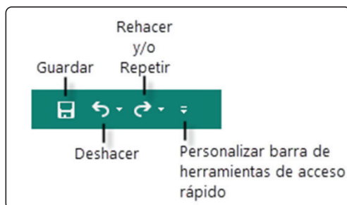
Figura 1.7. La barra de herramientas de acceso rápido (Publisher 2016)
