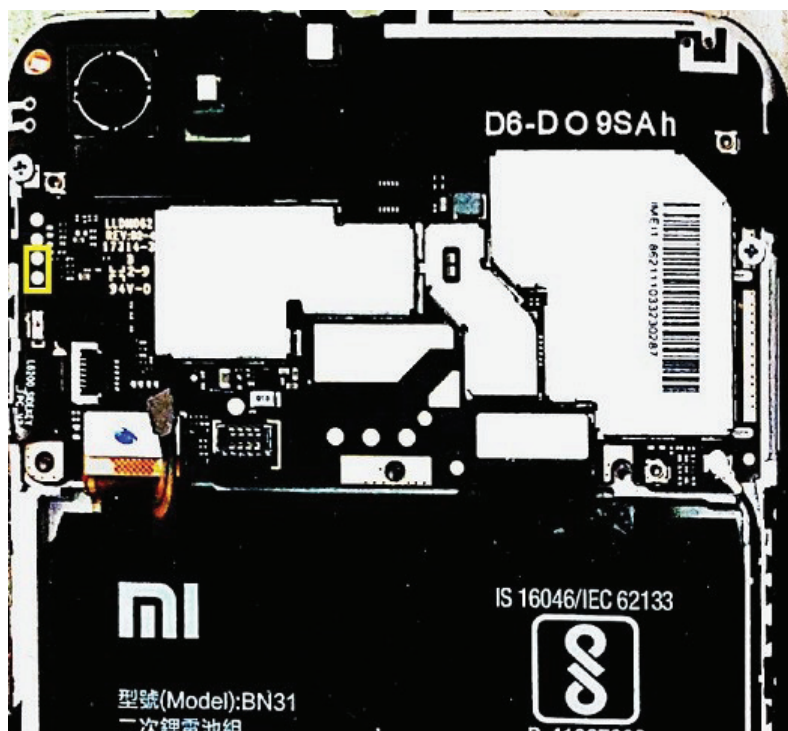
Ilustración 10. Ejemplo de los puertos que deben ser cortocircuitados para establecer el modo EDL en un dispositivo Xiaomi Note 5A. Fuente: Magnet Forensics.
